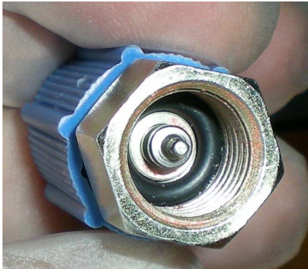
アキュムレータ側(ムシの反対側が見える)
