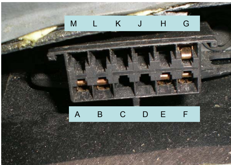
フィエロのALDLコネクタピンアサイン
