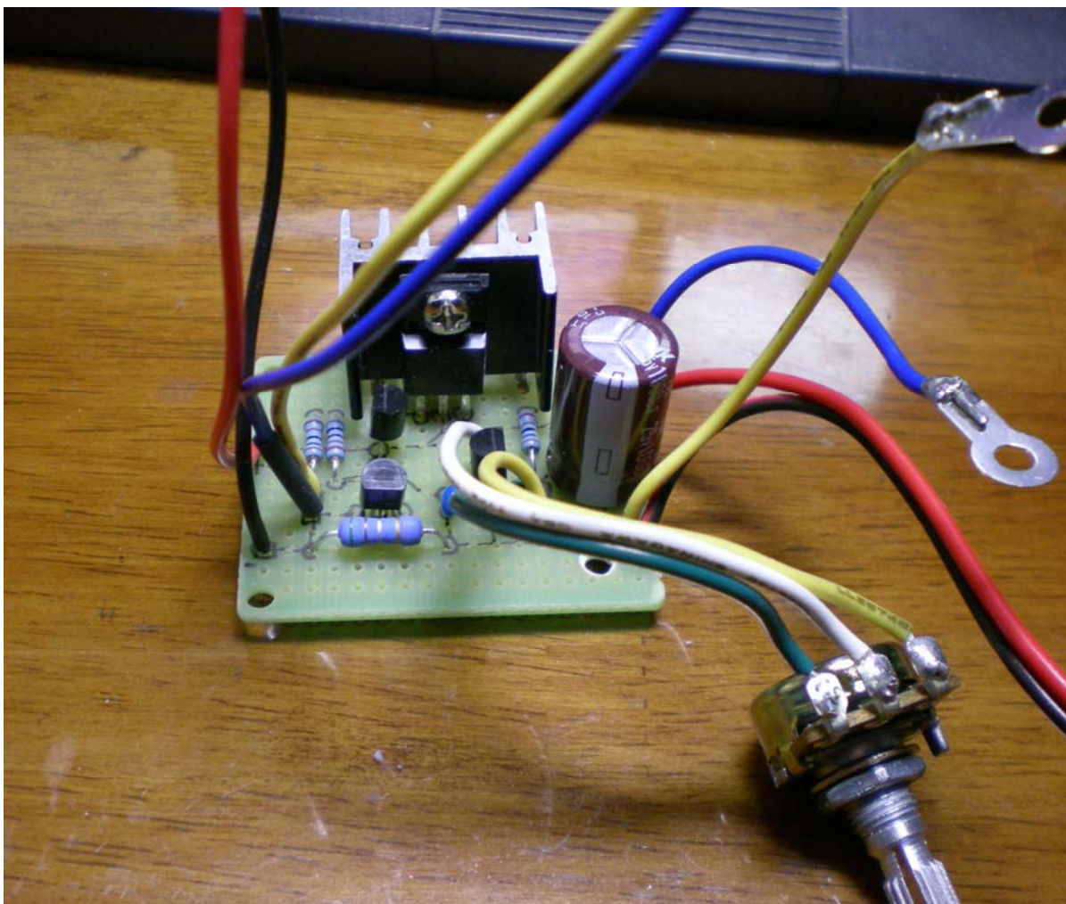
基板
