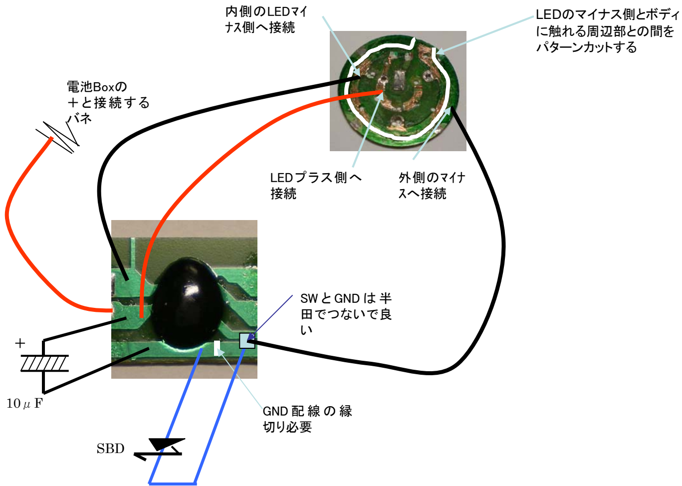
点滅回路の配線
