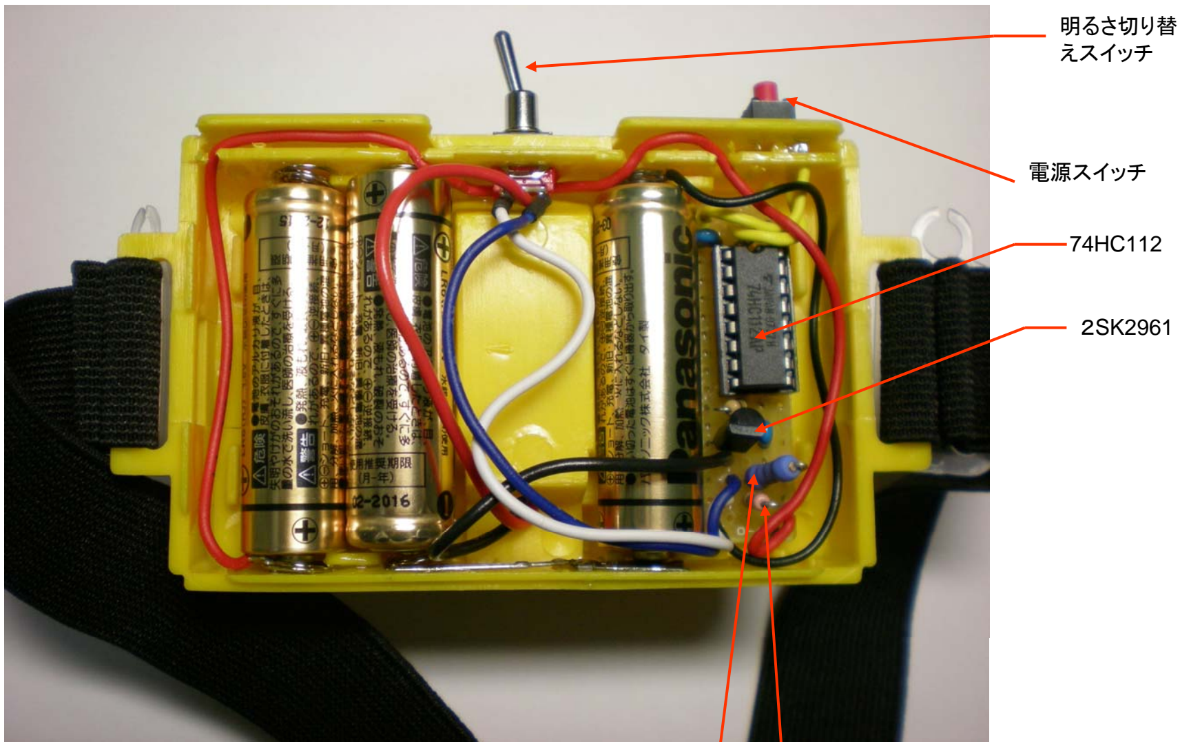
オルタネートスイッチ回路
