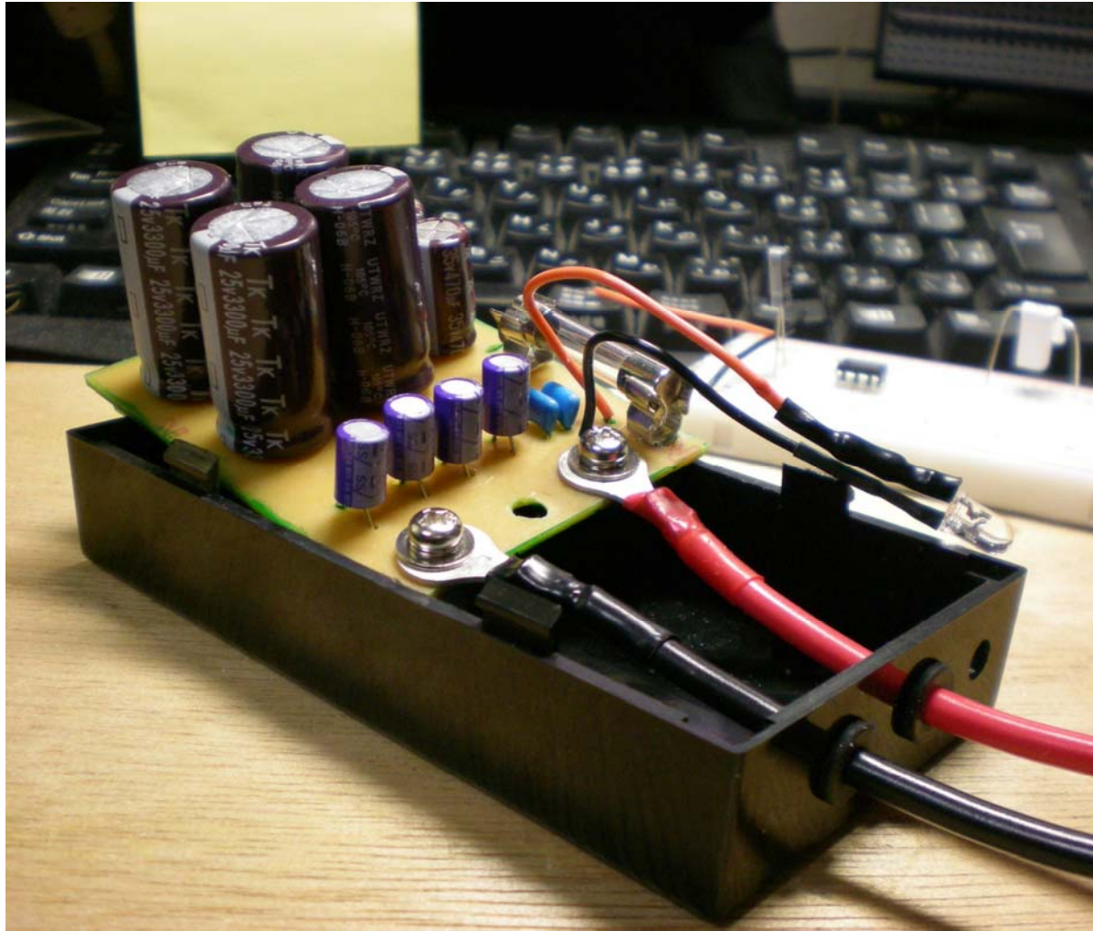
コンデンサー固定前の状態
