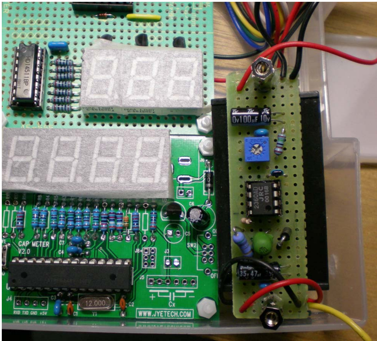
電池Box裏の昇圧回路
