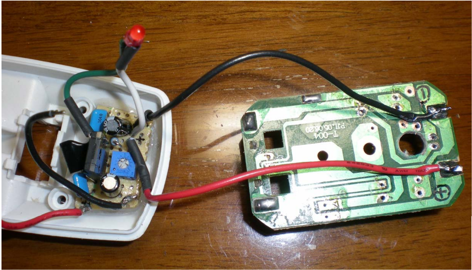
ケースに回路を組み込み中
